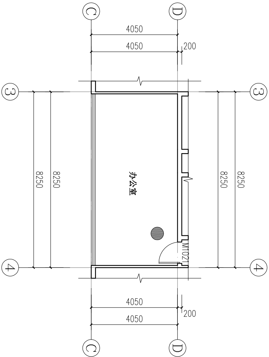
五层原建筑图二 1:100
