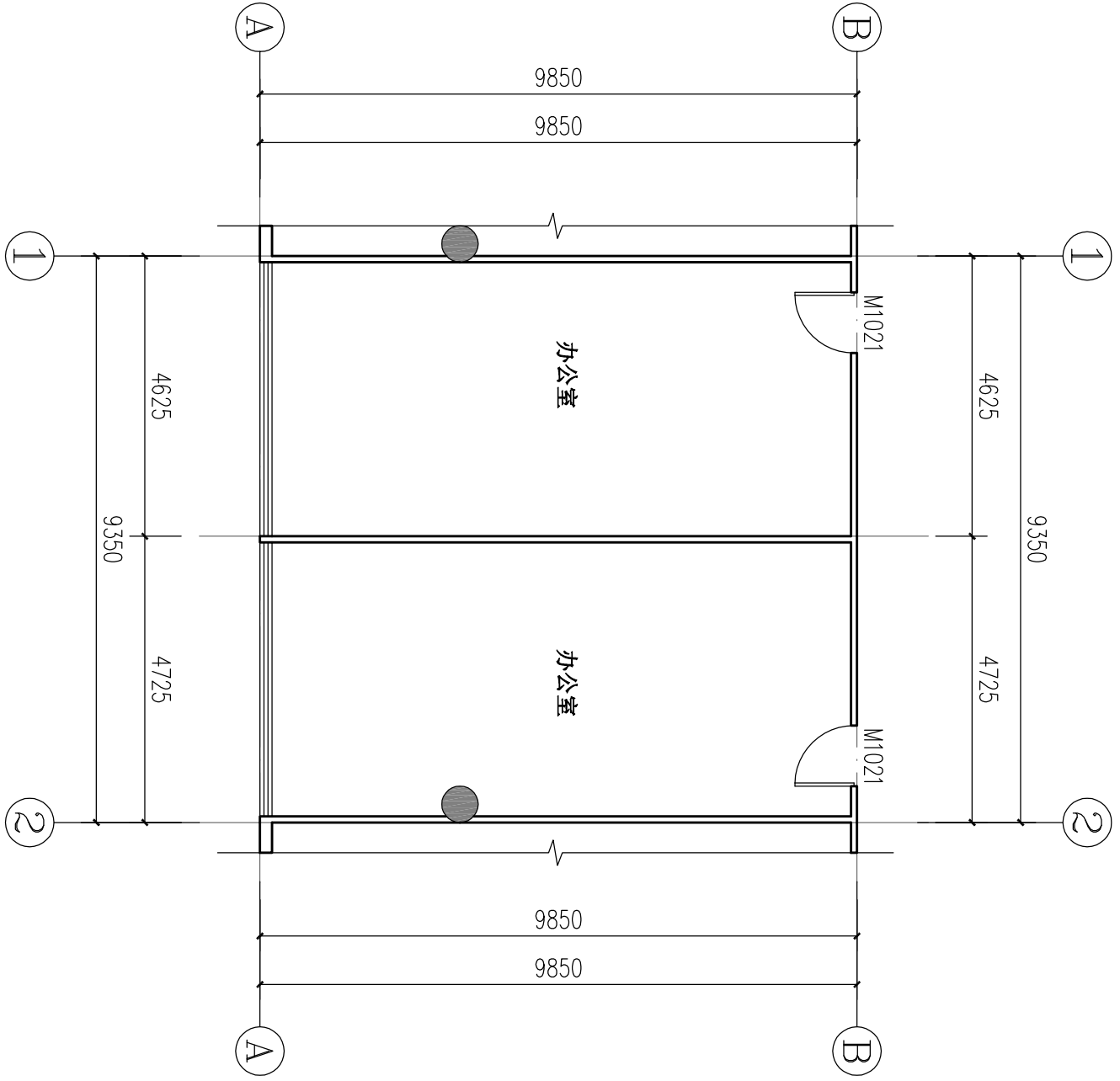
五层原建筑图一 1:100
