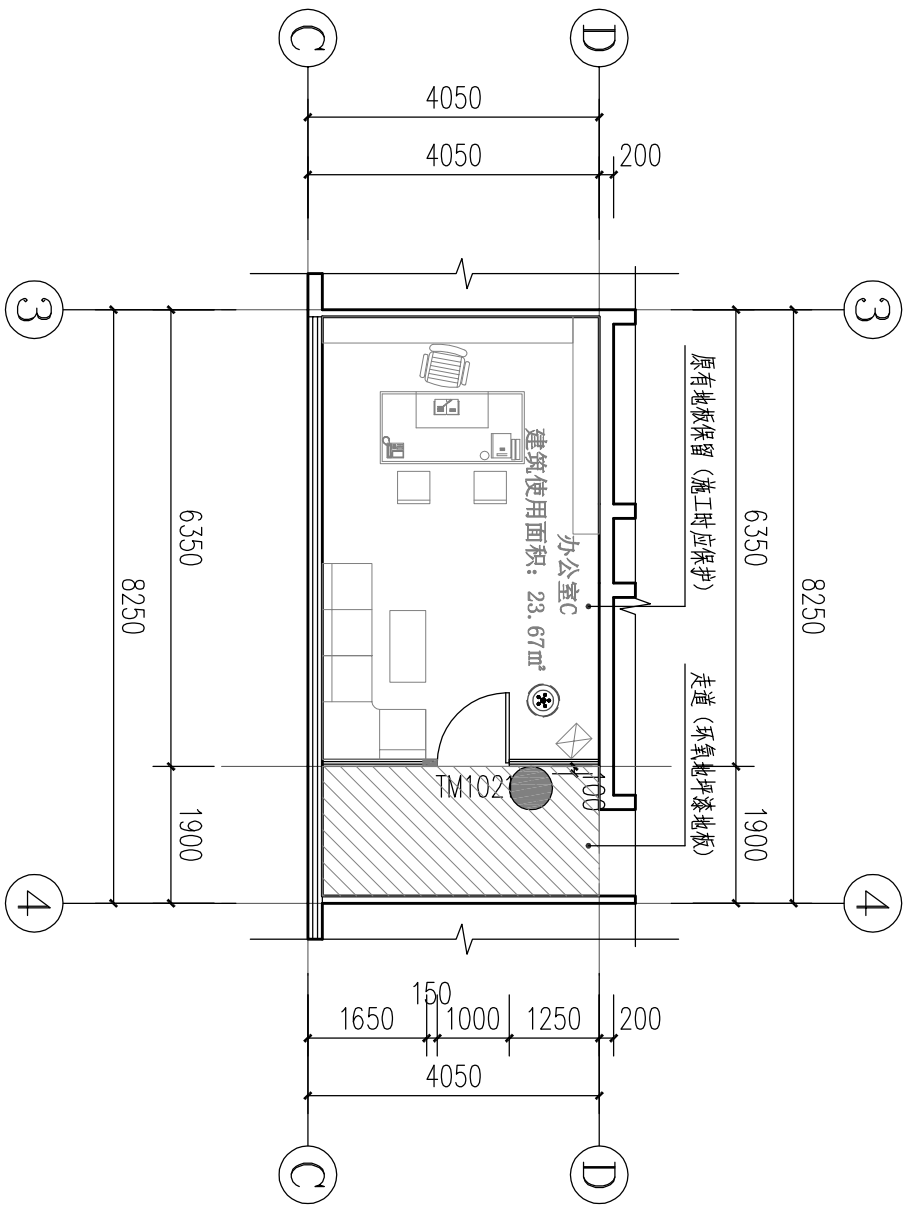
地面铺装图二 1:100
