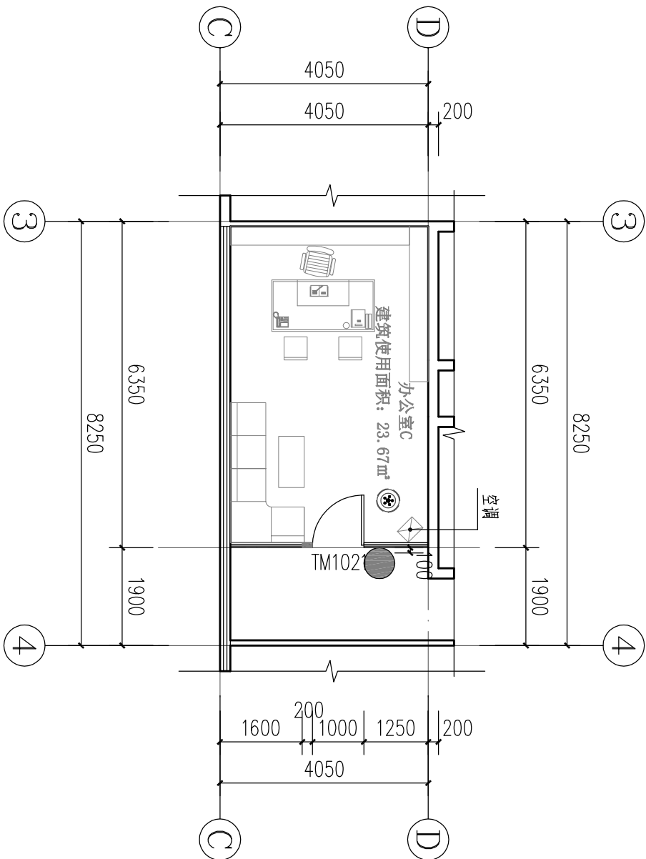
平面布置图二 1:100
